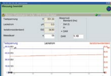
Měření izolace
